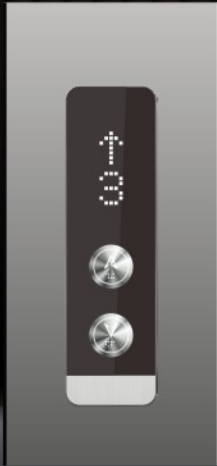
HD-LOP29 选配 面板: 铝合金边框+玻璃面板 图示显示板型号: ZT-D5-3.2 尺寸: 180mm*58mm*12mm
